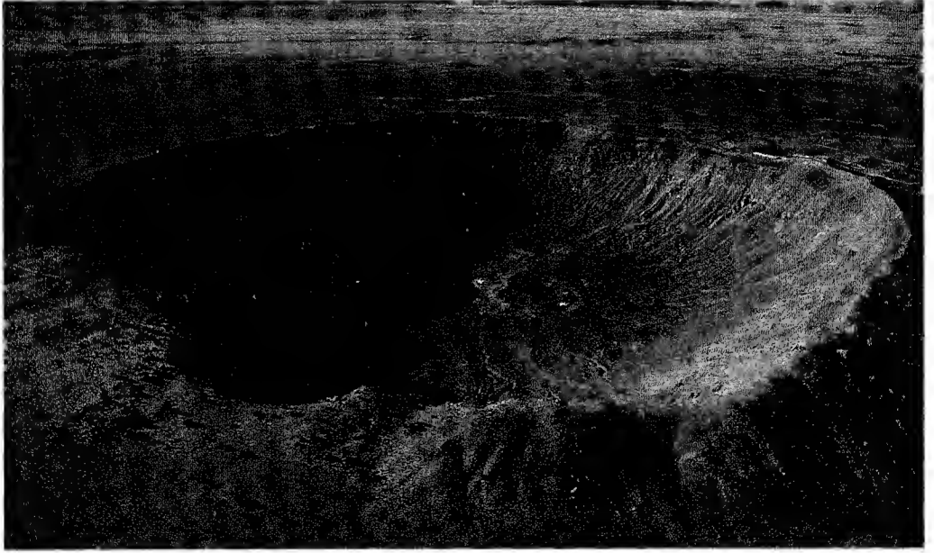
فجوة ضخمة (يبلغ طول قطرها 32 كلم تقريباً) تكونت من جراء ارتطام نيزك بأرض ولاية أريزونا
